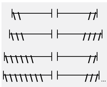
Esquemas de tope para contraventanas articuladas en tijera, resumen
